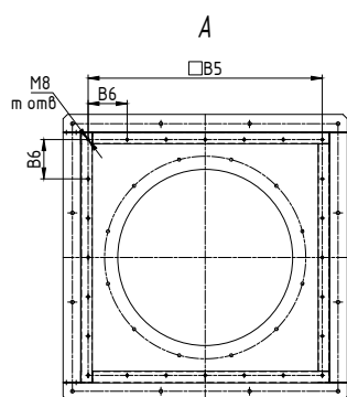
Стакан СТВ... вид снизу
