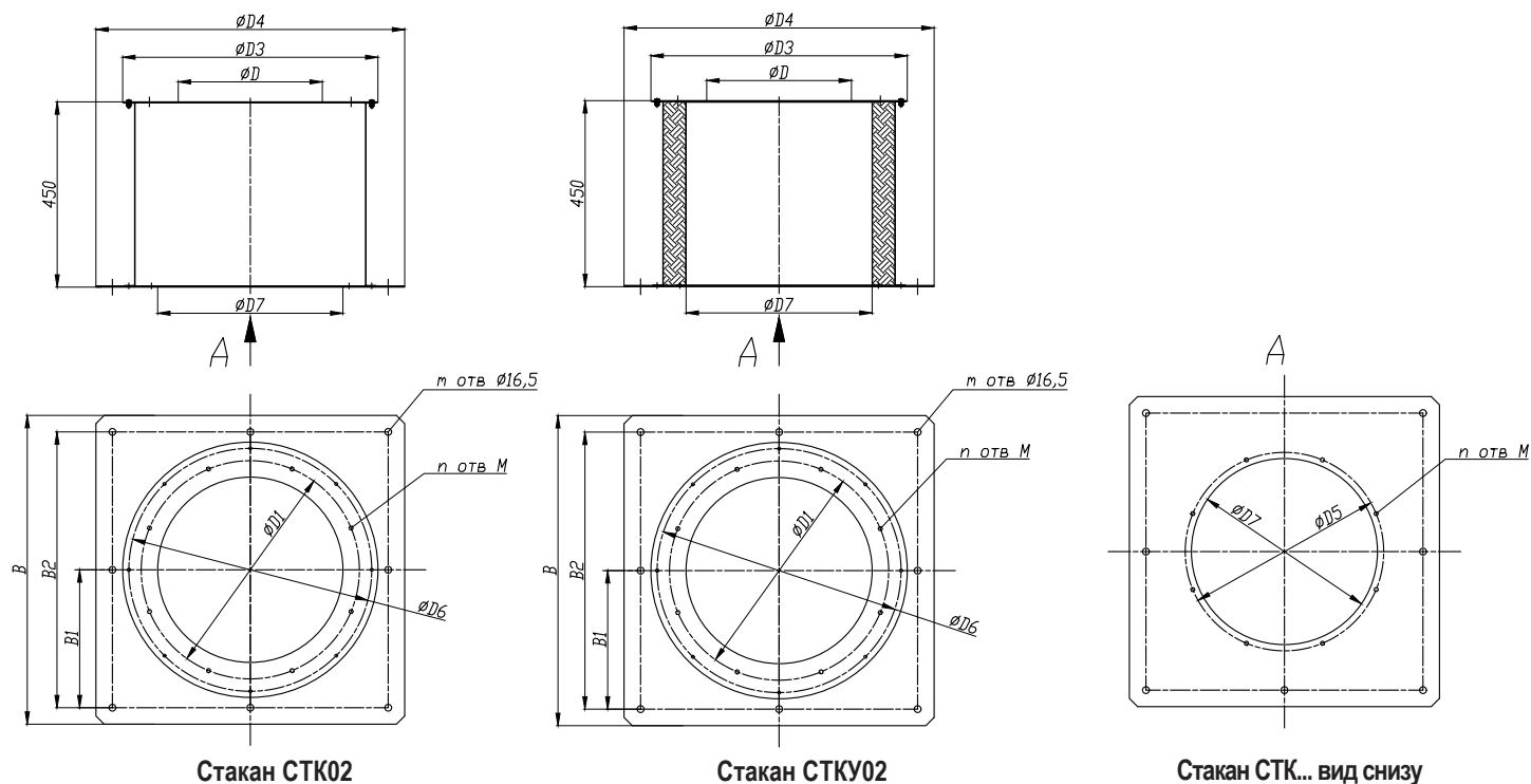
Размеры и массовые характеристики круглых стаканов для дефлектора с квадратным основанием
