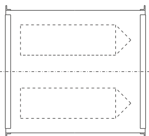
Пластиновый шумоглушитель с обтекателем
