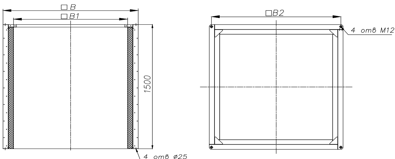
Размеры и массовые характеристики Базы UFW для стаканов ВКР-Ф
