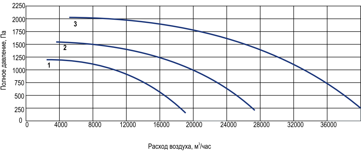
ВЕНТИЛЯТОР ВКП-Р (РАДИАЛЬНЫЙ ВЕНТИЛЯТОР ДВУХСТОРОННЕГО ВСАСЫВАНИЯ)
