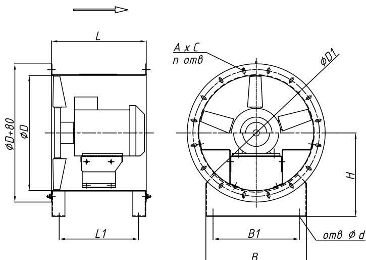
Размеры Вентиляторов НАПОР
