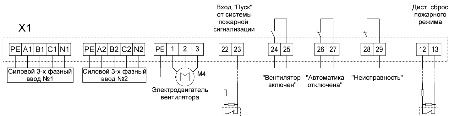
ТИПОВАЯ СХЕМА ВНЕШНИХ ПОДКЛЮЧЕНИЙ ШКАФОВ VAD-D
