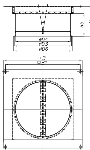
Клапан обратный для ВКР-Ф
