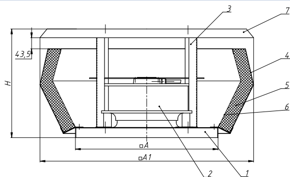
Вентилятор VKVT(S)
