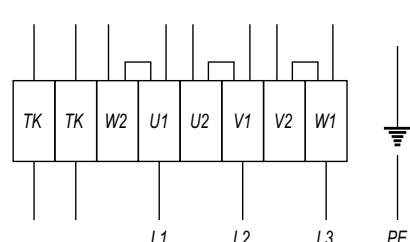
Схема подключения трехфазного двигателя вентилятора VKV
