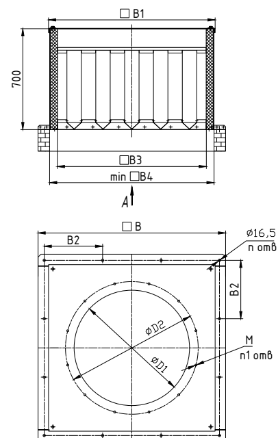
Стакан СТКУ-Ш
