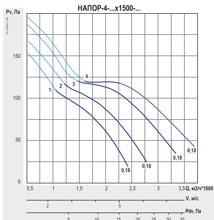
Диаграммы характеристик Вентиляторов НАПОР
