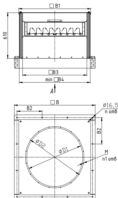
Стакан СТКУ-ПВ
