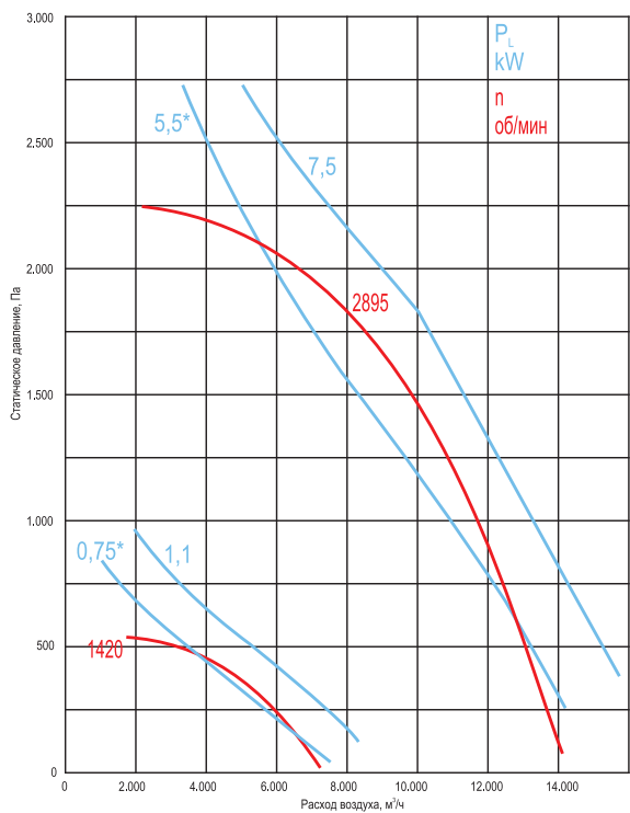
ВКР-4,5-ДУ-С-...
