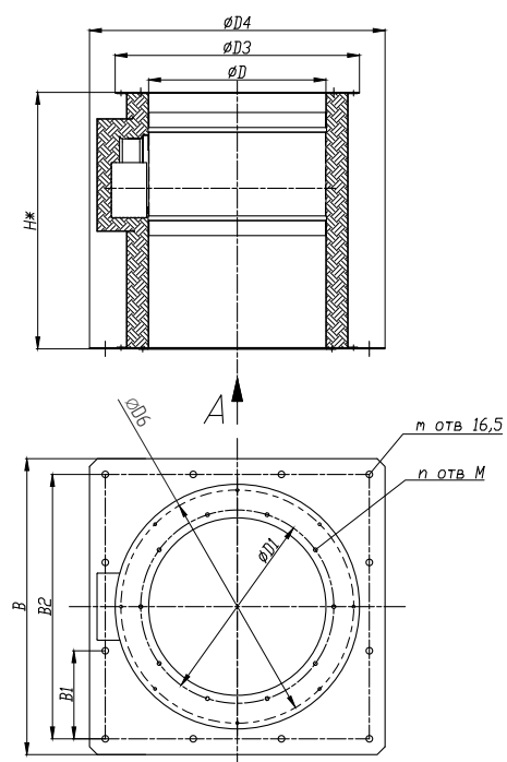
Стакан СТКУ-П02
