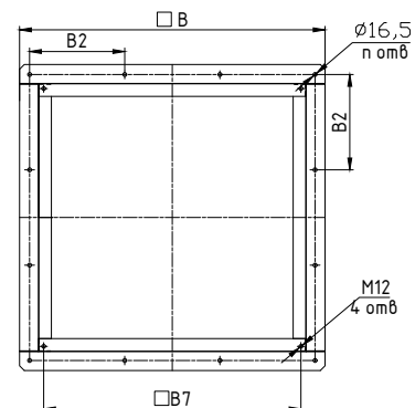
Стакан СТКУ-К
