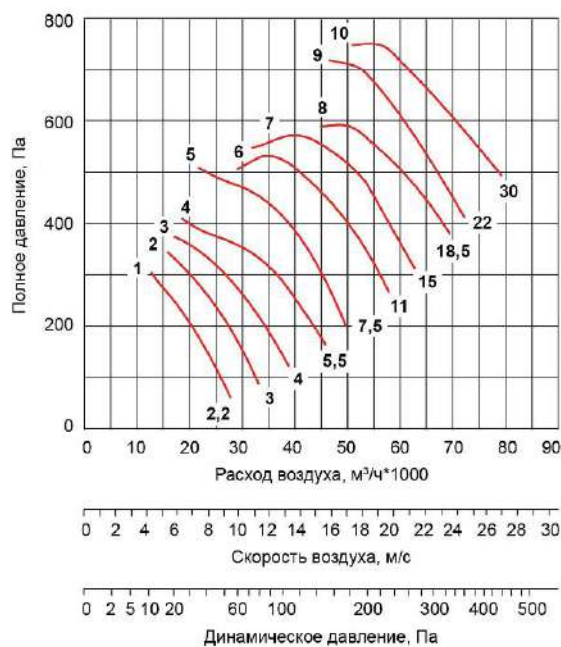
ВО-100-ДУ-.../1500-...
