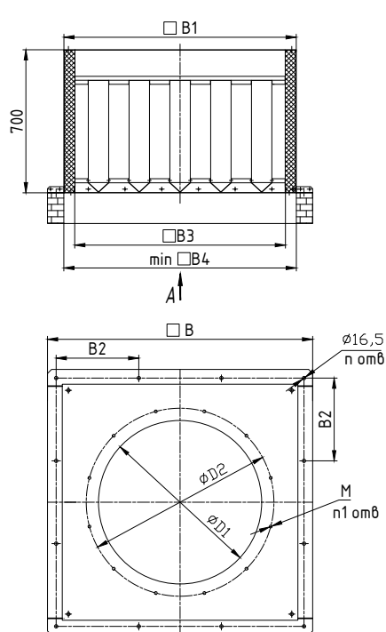
Стакан СТКУ-Ш
