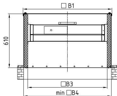
Стакан СТКВ-М
