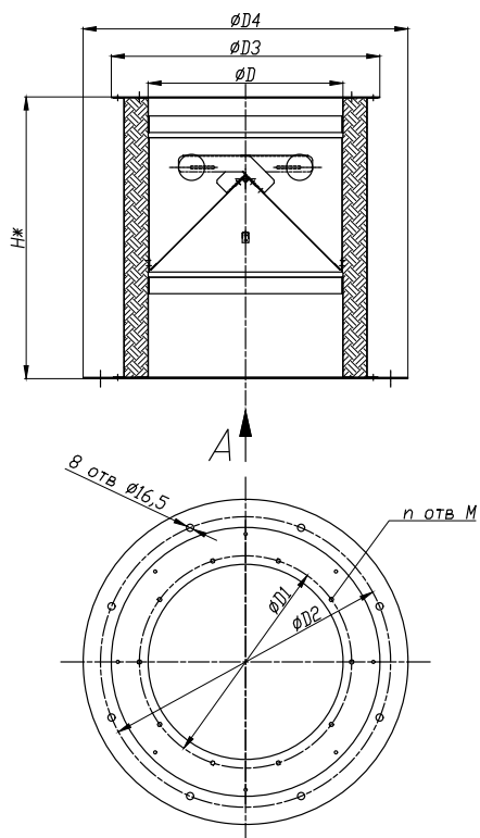
Стакан STKY-П01 приток
