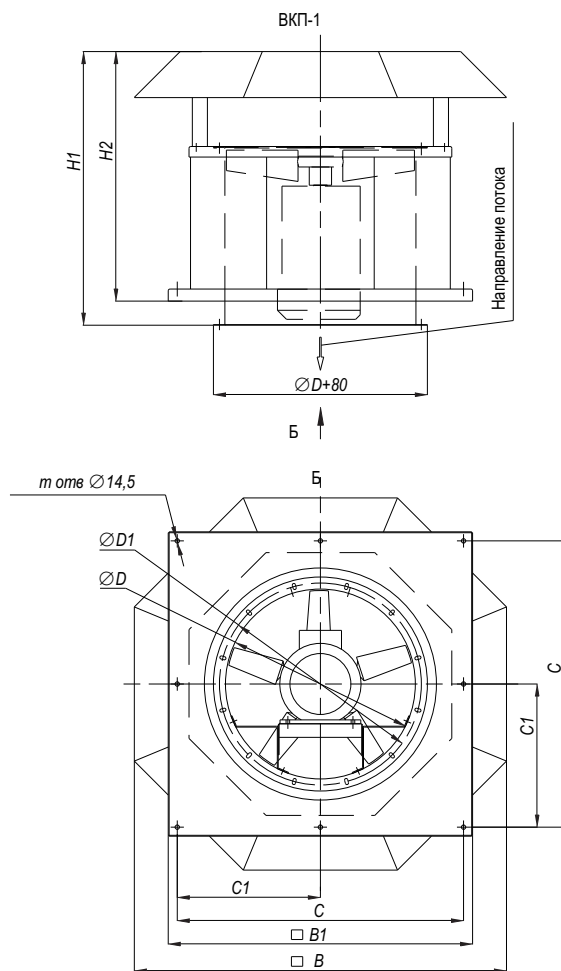
Размеры вентиляторов ВКП-0 / ВКП-1
