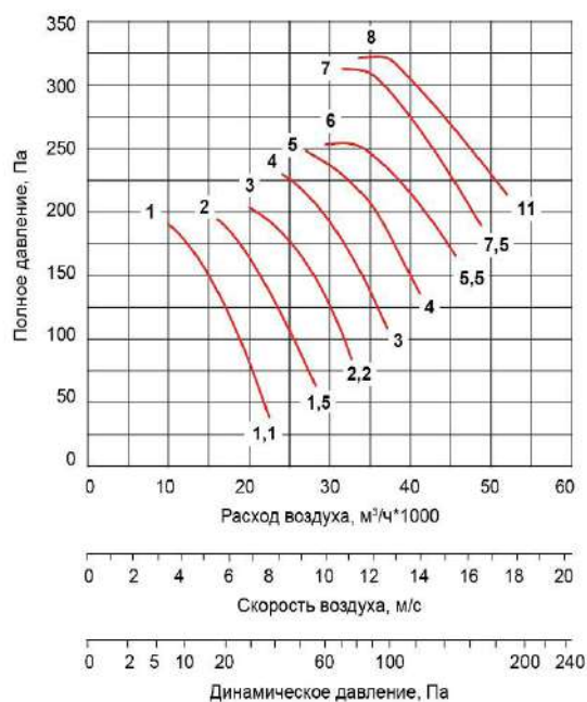
ВО-100-ДУ-.../1000-...
