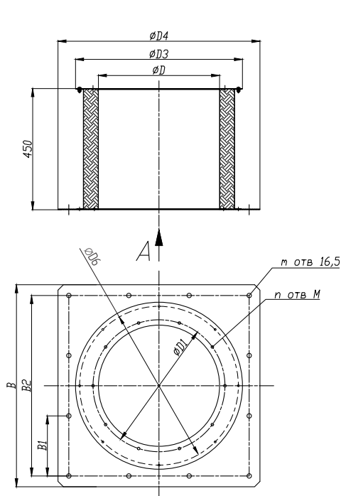
Стакан СТКУ02
