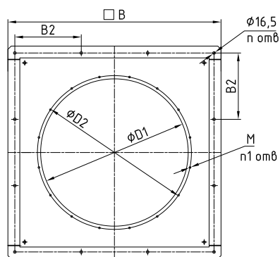
Стакан СТКВ-М
