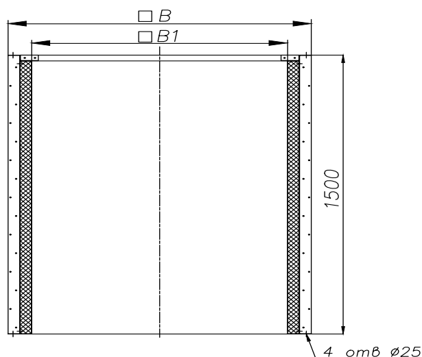
Размеры и массовые характеристики База UFW для стаканов ВКР-Ф
