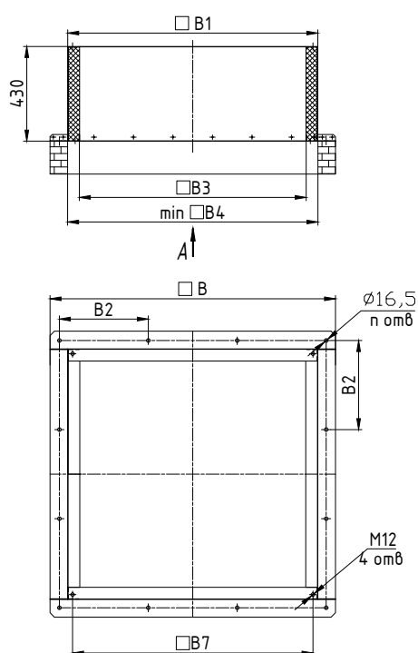
Стакан СТКУ-М
