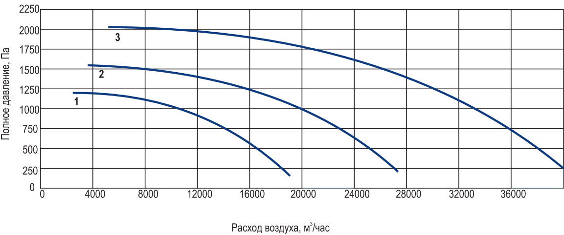
ВЕНТИЛЯТОР ВКП-РД (РАДИАЛЬНЫЙ ВЕНТИЛЯТОР ДВУХСТОРОННЕГО ВСАСЫВАНИЯ)
