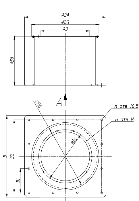
Стакан СТК02
