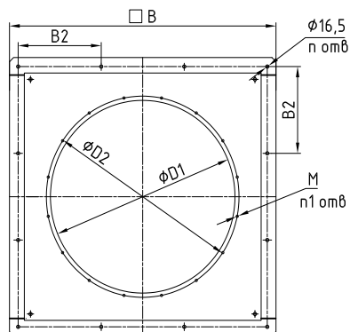
Стакан СТКУ-М
