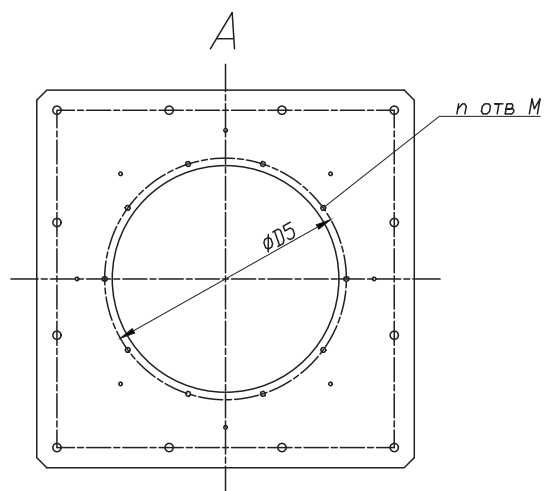
Стакан СТУ...- вид снизу
