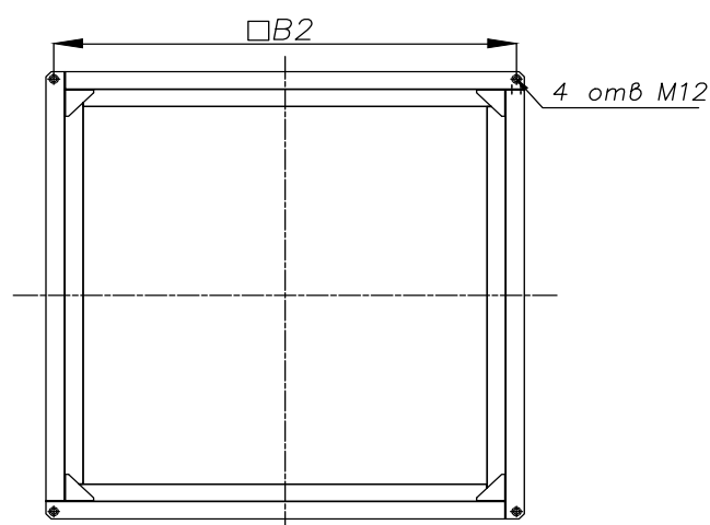
Размеры и массовые характеристики База UFW для стаканов ВКР-Ф
