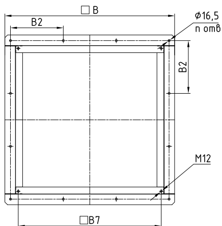
Стакан STKB-M
