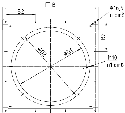
Стакан STKY-P
