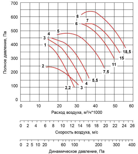
ВО-090-ДУ-.../1500-...
