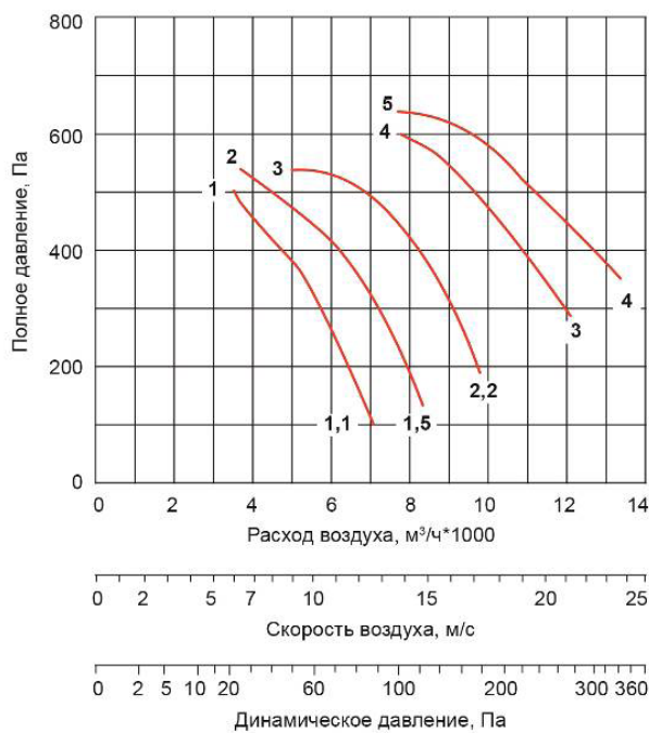
ВО-045-ДУ-.../3000-...
