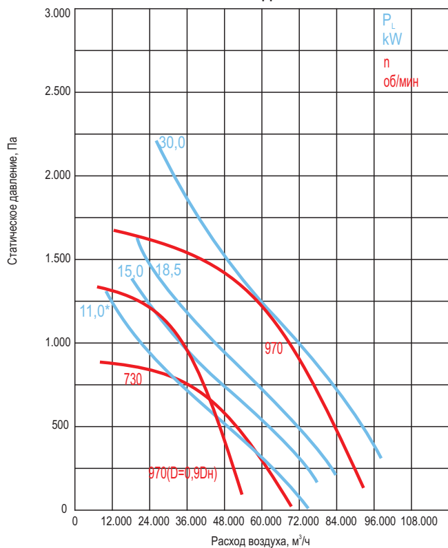
ВКР-11-ДУ-Ф-...
