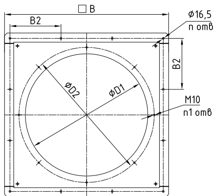
Стакан STKB-M
