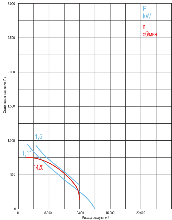
ВКР-5-ДУ-С-...
