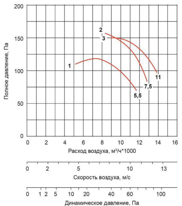
ВО-063-ДУ-.../1000-...
