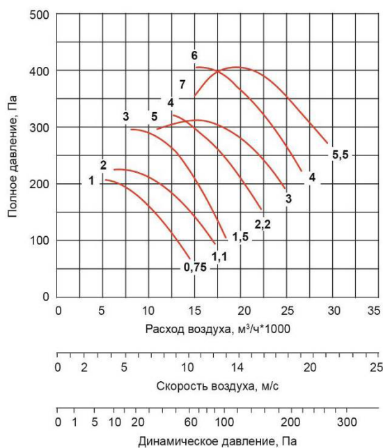
ВО-071-ДУ-.../1500-...
