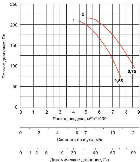
ВО-050-ДУ-.../1500-...
