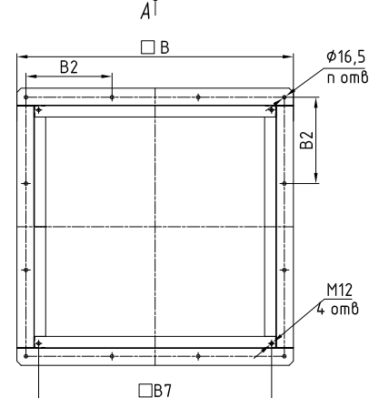
Стакан STKU-K
