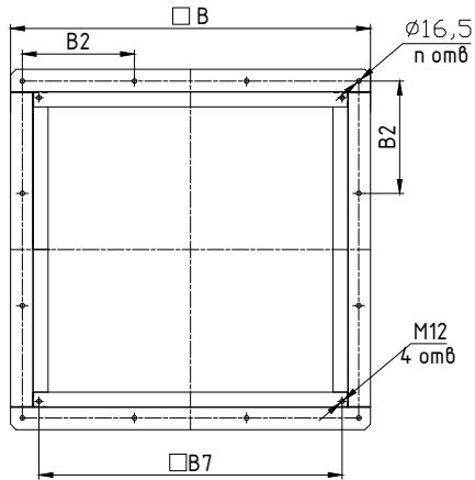
Стакан STKU-M
