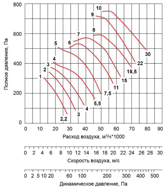
ВО-100-ДУ-.../1500-...
