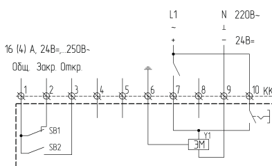
Схема подключения клапана КДМ с ЭМ -вар1
